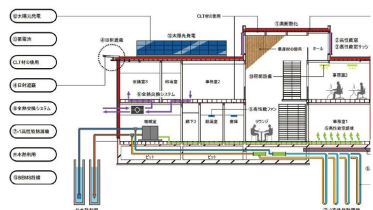
太陽光発電と蓄電池によりライフライン遮断時も電気の利用が可能
